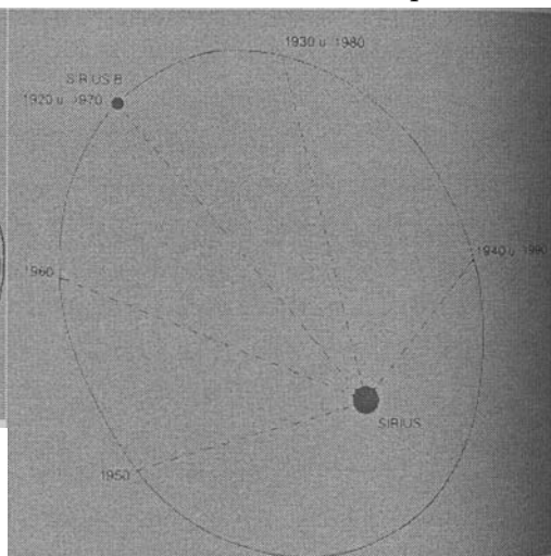
Obr. 49: Moderní astronomický diagram oběžné dráhy Sิริuse B, který zobrazuje jeho polohu v konkrétních letech.
