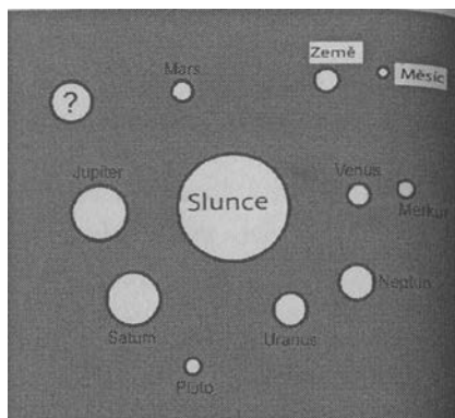
Obr. 29: Sluneční soustava - pro srovnání: tak, jak ji známe i dnes a s další, nám neznámou planetou.
