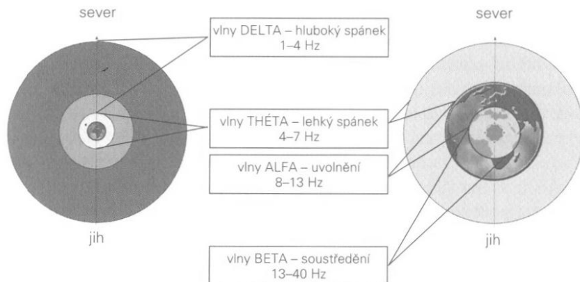
Obr. 3.18 Fyzikální sférické segmenty Země a příslušné stavy mentálního vědomí.
