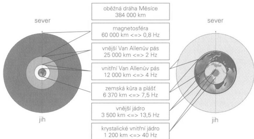
Obr. 3.16 Vzdálenosti jednotlivých sférických polí od středu Země a jejich příslušné elektrické frekvence.
